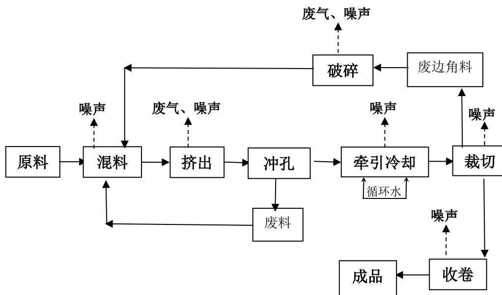
图2 项目运营期生产工艺流程及产污环节示意图
