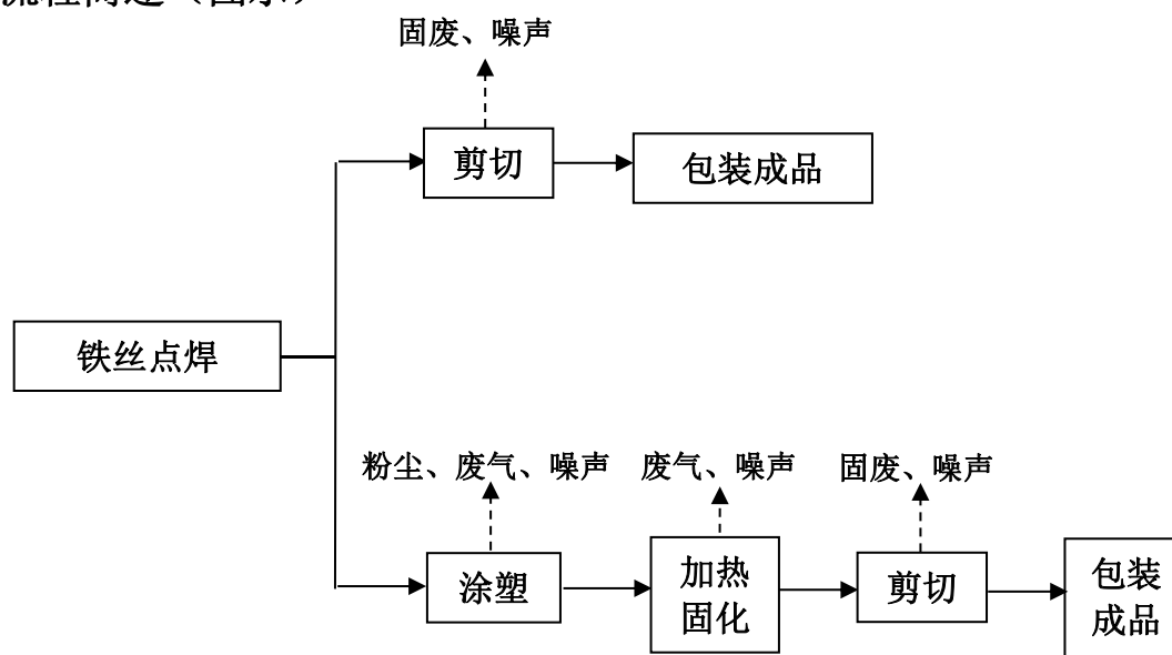
图1 项目营运期生产工艺流程及产污环节图
